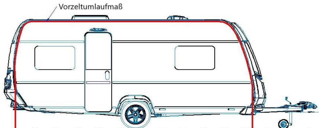
Maßschema für Vorzeltumlaufmaß
